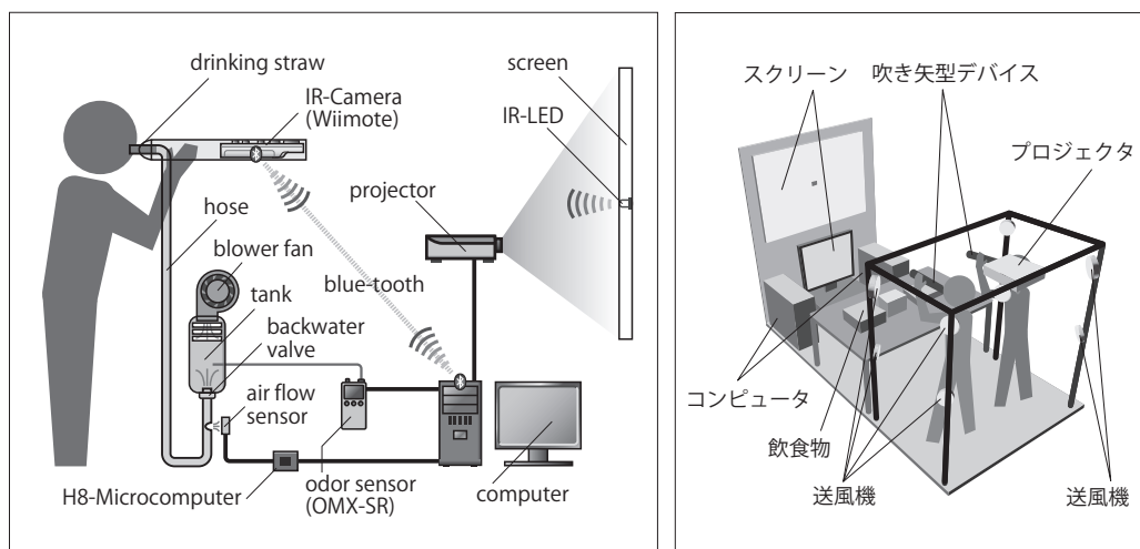
図1-6 「La flèche de l'odeur」のシステム構成図（小坂研究室提供）
